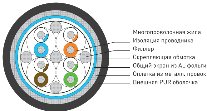
Рис. 1 — Конструкция кабеля SF/UTP (количество жил 4x2x19)
